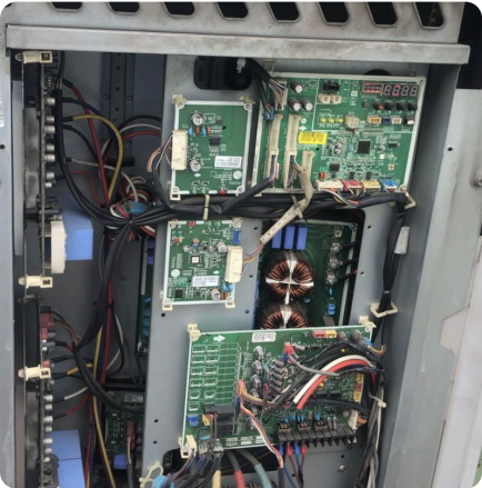
Kiểm tra board dàn nóng LG Multi V
