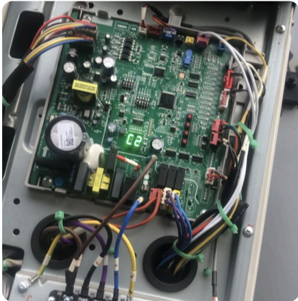
Đọc mã lỗi board Samsung DVM
