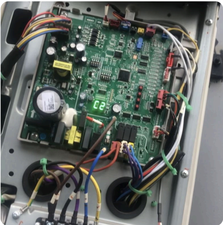
读取三星 DVM 电路板故障代码
