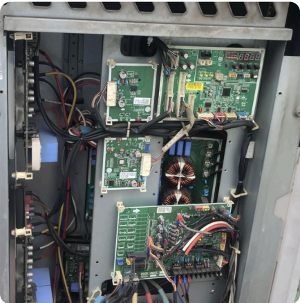
检测 LG Multi V 室外机电路板
